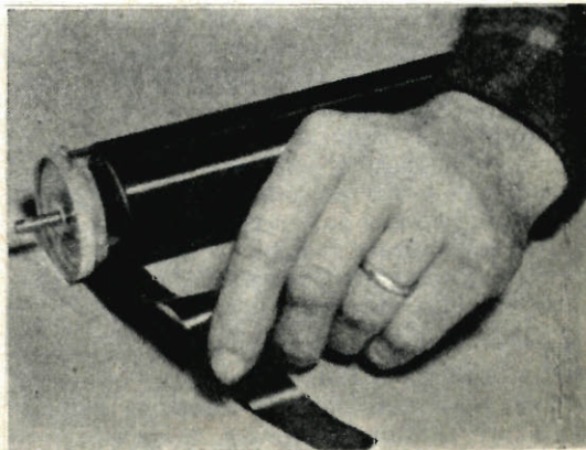
Fig. 12 - Si completi il lavoro con una striscia di nastro isolante di carta gommata.
