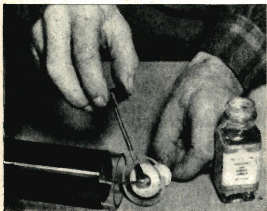
Fig. 13 - Occorre stendere uno strato di vernice isolante sull'isolatore.
