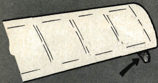
Fig. 5 - Il pareggio delle incidenze si raggiunge facilmente aggiungendo un alettone di cartoncino o di celluloido all'estremità dell'ala che si abbassa durante la virata.
