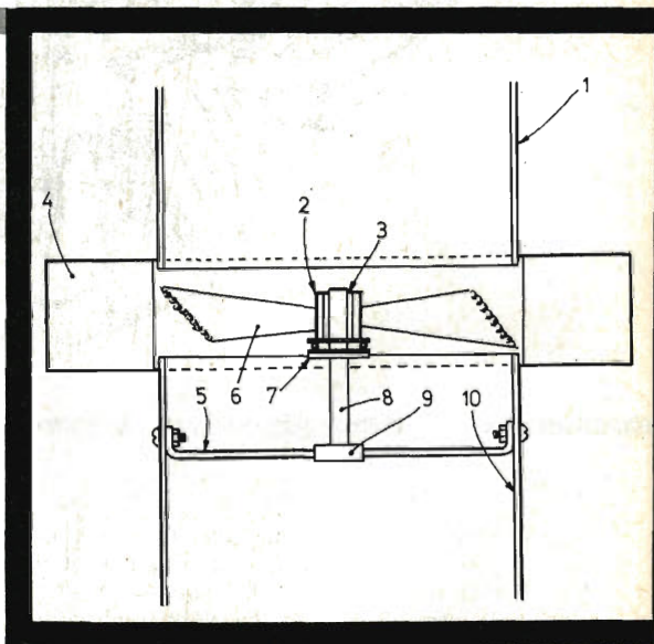
Fig. 2 - Vista in sezione del complesso: 1 - tubo superiore. 2 - mozzo e boccola di bronzo. 3 - perno. 4 - pala esterna. 5 - staffe di sostegno della struttura. 6 - pala interna. 7 - flangia sostegno ventola saldata sul perno (sopra il cuscinetto reggispinta). 8 - perno. 9 - flangia sostegno perno saldata sul medesimo. 10 - tubo inferiore.
