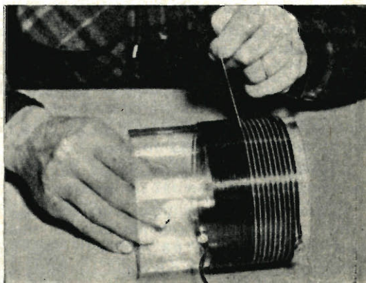
Fig. 16 - Si possono spaziare le spire della bobina più larga avvolgendo uno spago tra i fili.
