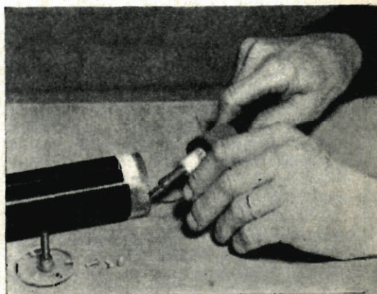
Fig. 10 - Si tenga fermo temporaneamente il filo libero mentre si salda al suo posto la giunzione.
